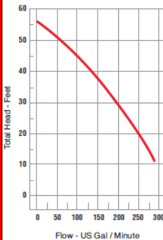
SL-500 (P30CS)
