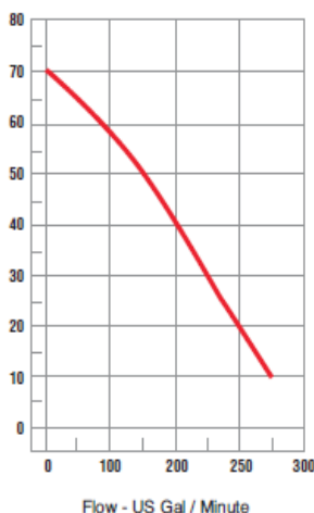
SL-750 (P40CS)
