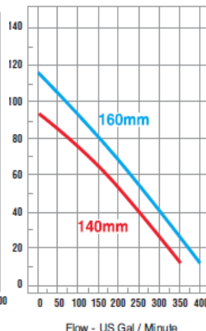
SL-1000 (P50CS)
